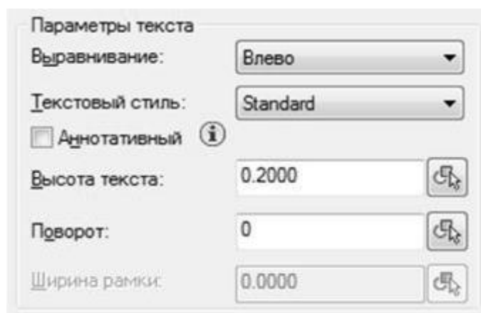
Рис. 5.11. Розділ „Параметры текста” діалогового вікна команди „ATTDEF (Атрибут)”
