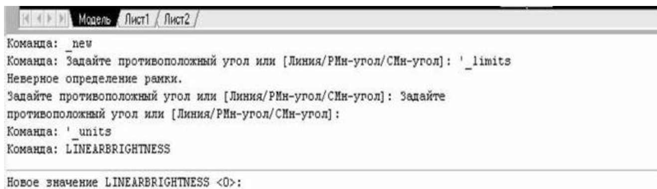
Рис. 2.2. Вікно команд
