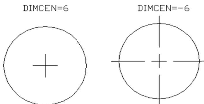
Рис. 6.16. Застосування змінної DIMCEN для керування розміром маркера або позначення осевих ліній
